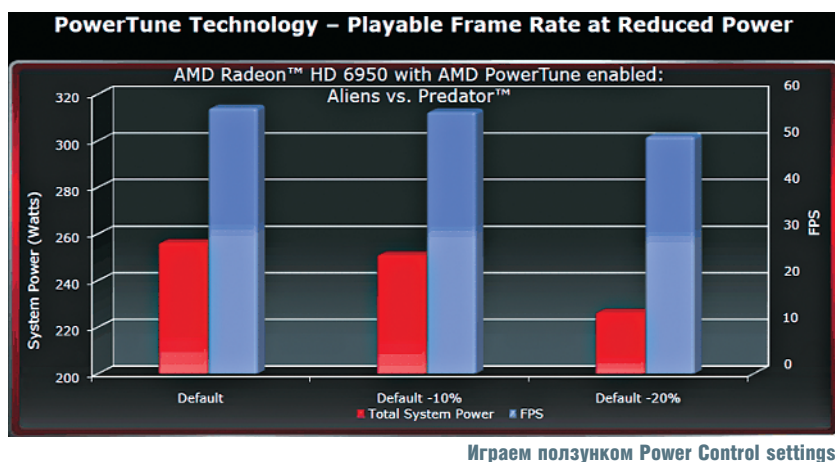
Играем ползунком Power Control settings
