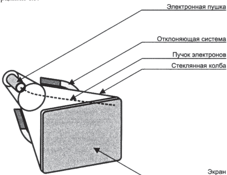
Устройство электронно-лучевой трубки
