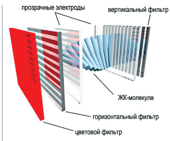
Устройство субпикселя ЖК-матрицы
