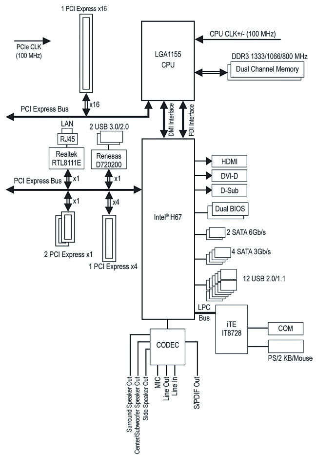
Блок-схема материнской платы GA-H67MA-UD2H
