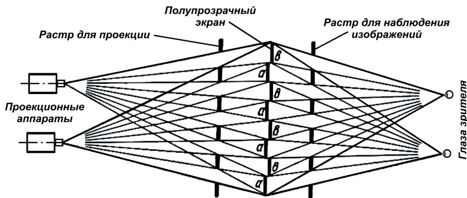
Рис. 4. Схема растровой стереопроекции на просветный экран
