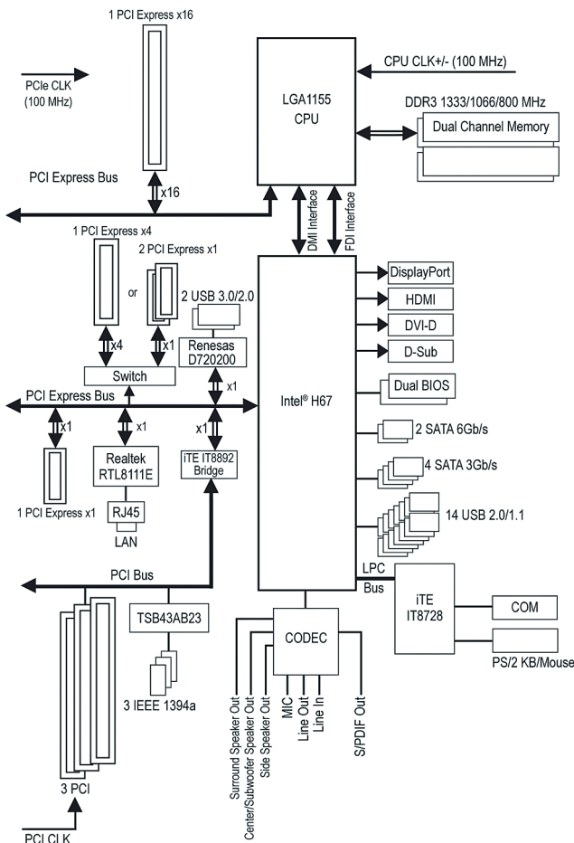
Блок-схема материнской платы GA-H67A-UD3H
