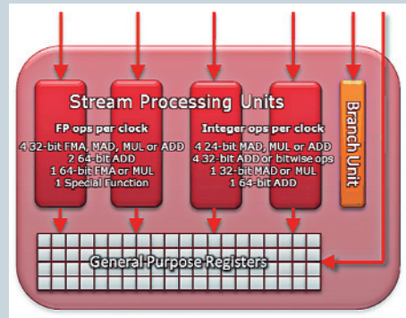
Блок-схема потокового процессора
