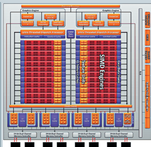
Углубленная блок-схема графического процессора Cayman
