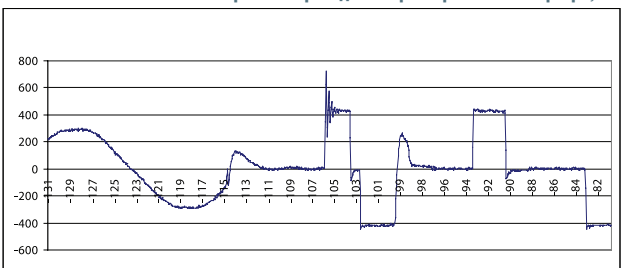
Прямая переходная характеристика инвертора, 8,7 мс
