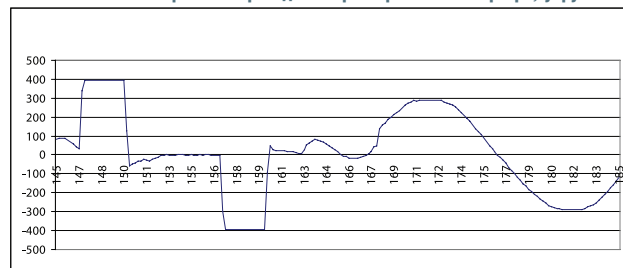
Типичная обратная переходная характеристика инвертора, подробно
