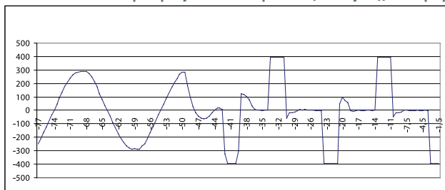
Прямая переходная характеристика инвертора, 8 мс
