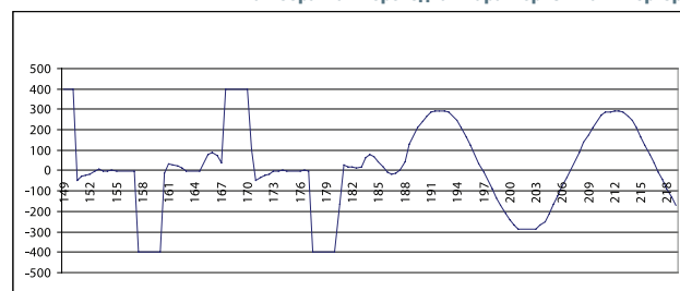
Типичная обратная переходная характеристика инвертора, укрупненно
